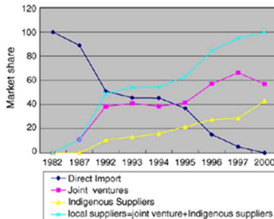
شکل ۴- سهم بازار کلیدهای خودکار در چین
