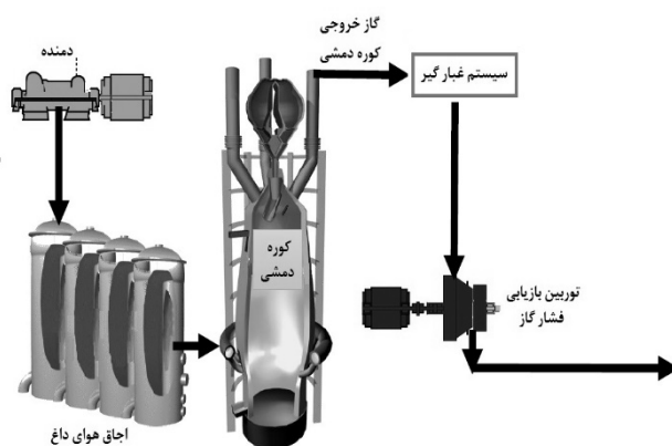
شکل 19: توربین بازیابی فشار گاز بالای کوره دمشی (TRT)
