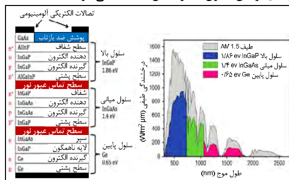
شکل 9: ساختمان یک نمونه سلول فتوولتائیک چندپیوندی [25]
