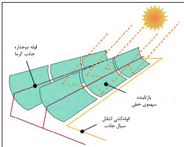
شکل 13: طرحواره یک کلکتور سهموی خطی
